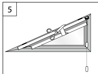
WANDWINKEL FÜR FD SLOPE 3
