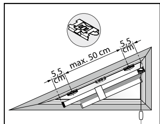
DECKENCLIP FÜR FD SLOPE 3 CEILING CLIP FOR FD SLOPE 3 – CLIP PLAFOND POUR FD SLOPE 3
